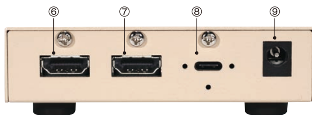
⑥ HDMI入力端子 ⑦ HDMI出力端子 ⑧ USB端子 ⑨ 電源入力端子
