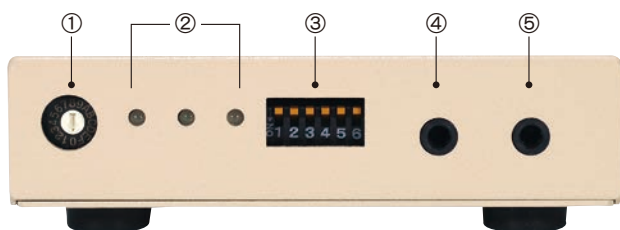
① EDID用ロータリスイッチ ② ステータスLED ③ 設定用DIPスイッチ ④ 音声出力端子 ⑤ 音声入力端子
